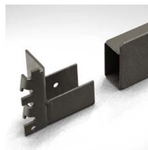
Držáky tvaru U k zavěšení trubkových profilů
