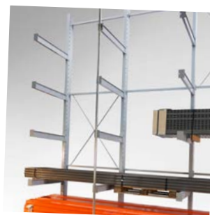
Ochranná tyč proti vypadnutí skladovaného materiálu
